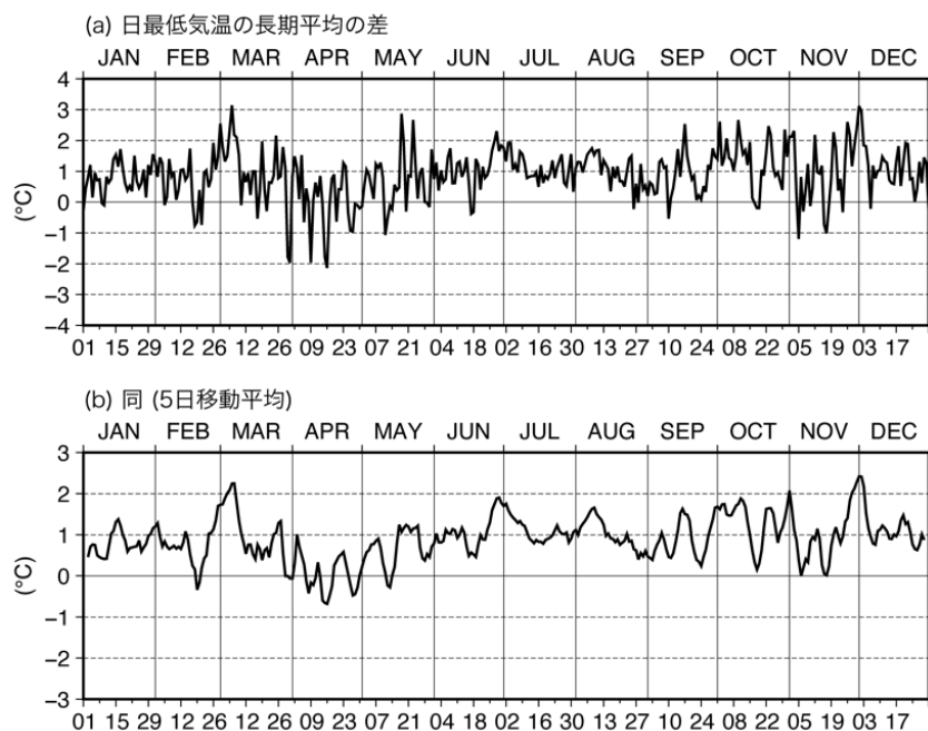
図 4: 京都府茶業研究所における日最低気温の長期変化傾向((1990-2021 年平均)-(1969-1989 年平均))
