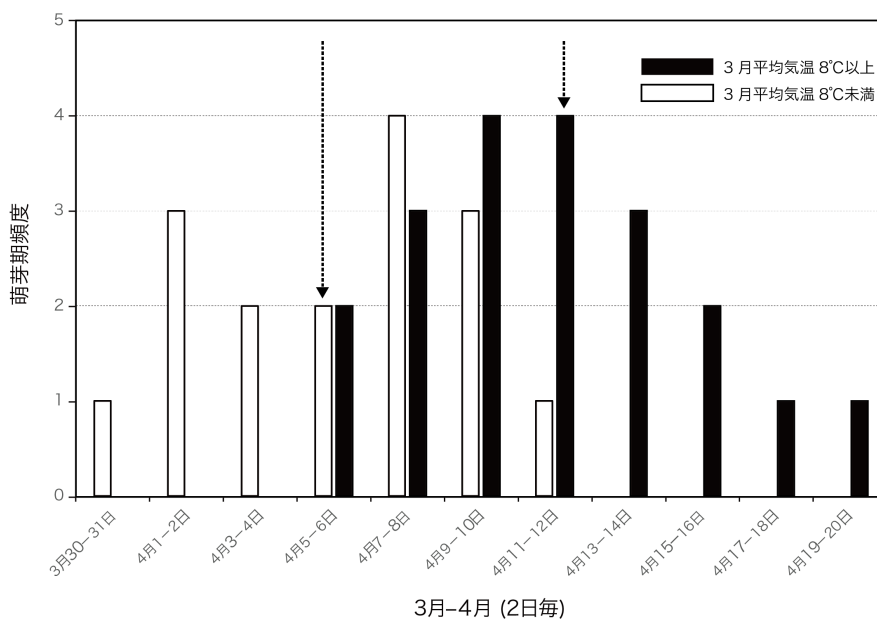
図 2: 京都府茶業研究所における一番茶の萌芽期の頻度分布(1987-2022 年) 3 月の平均気温 8°C 以上(16 年)であった萌芽期の中央値(破線)は 4 月 5 日 3 月の平均気温 8°C 未満(20 年)であった萌芽期の中央値(破線)は 4 月 11 日
