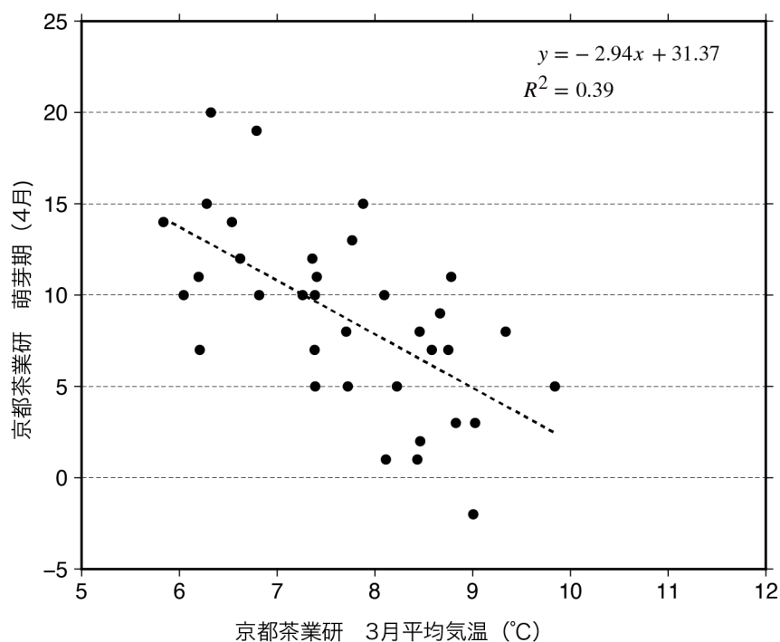
図 1: 京都府茶業研究所における一番茶の萌芽期(4 月のカレンダー日)と 3 月平均気温の 36 年間(1987 年-2022 年)における相関分布。縦軸の 0 は 3 月 31 日を、-5 は 3 月 26 日を示す。
