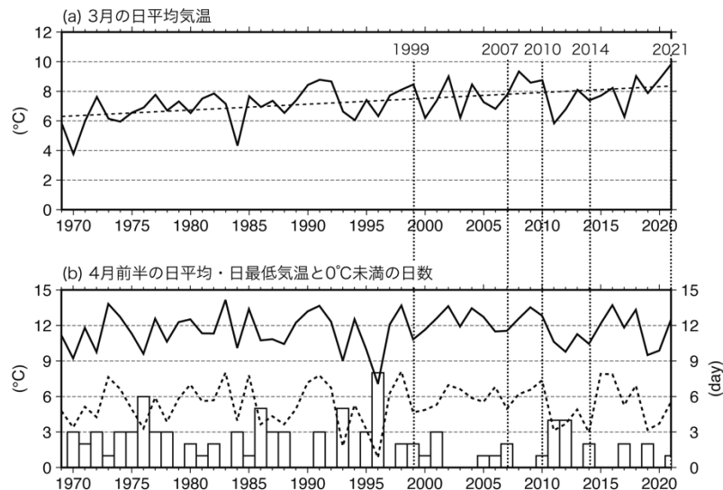
図 3: 京都府茶業研究所における 53 年間(1969 年-2021 年)の気温変化
