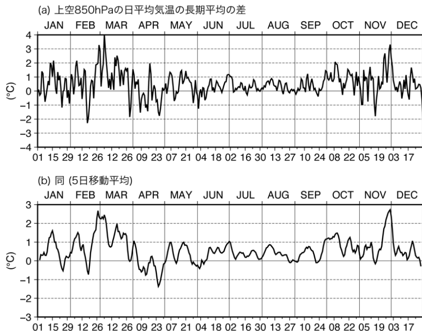
図 5: ヨーロッパ中期気象予報センター(ECMWF)の全球客観解析気象データ(ERA5)による京都府茶業研究所に最も近い格子点での 850 Pa(上空約 1500m)の気温の長期変化傾向((1990-2021 年平均)-(1969-1989 年平均))
