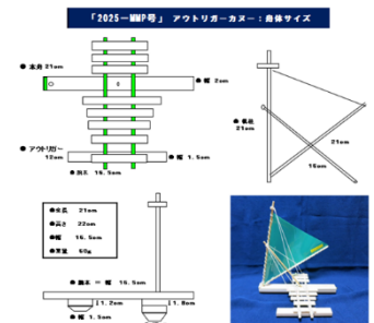
製作予定のアウトリガーカヌー模型
