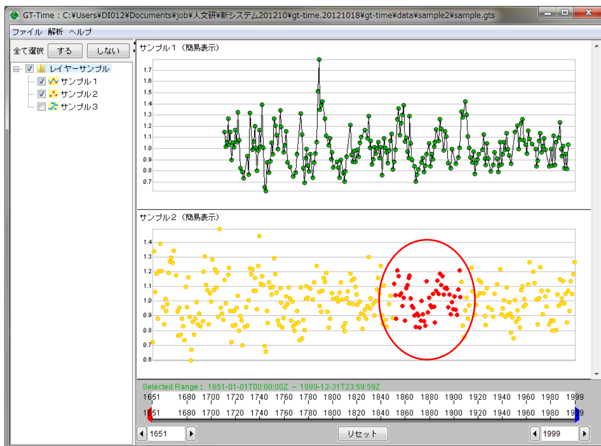
図 22-6 検索結果(ハイライト)
